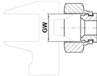
POMIAR GWINTU WEWNĘTRZNEGO
